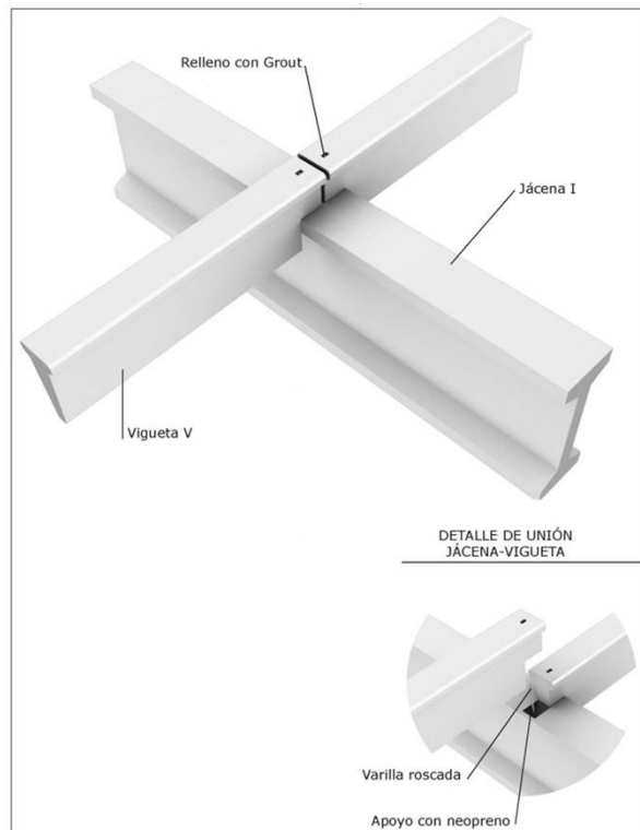
APOYO DE CORREAS EN V
