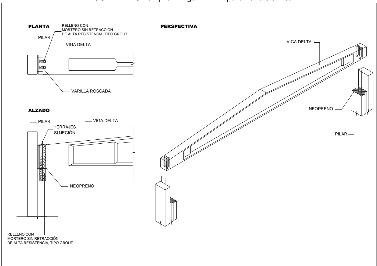
FIGURA 2.4. Unión pilar - viga DELTA para zona sísmica
