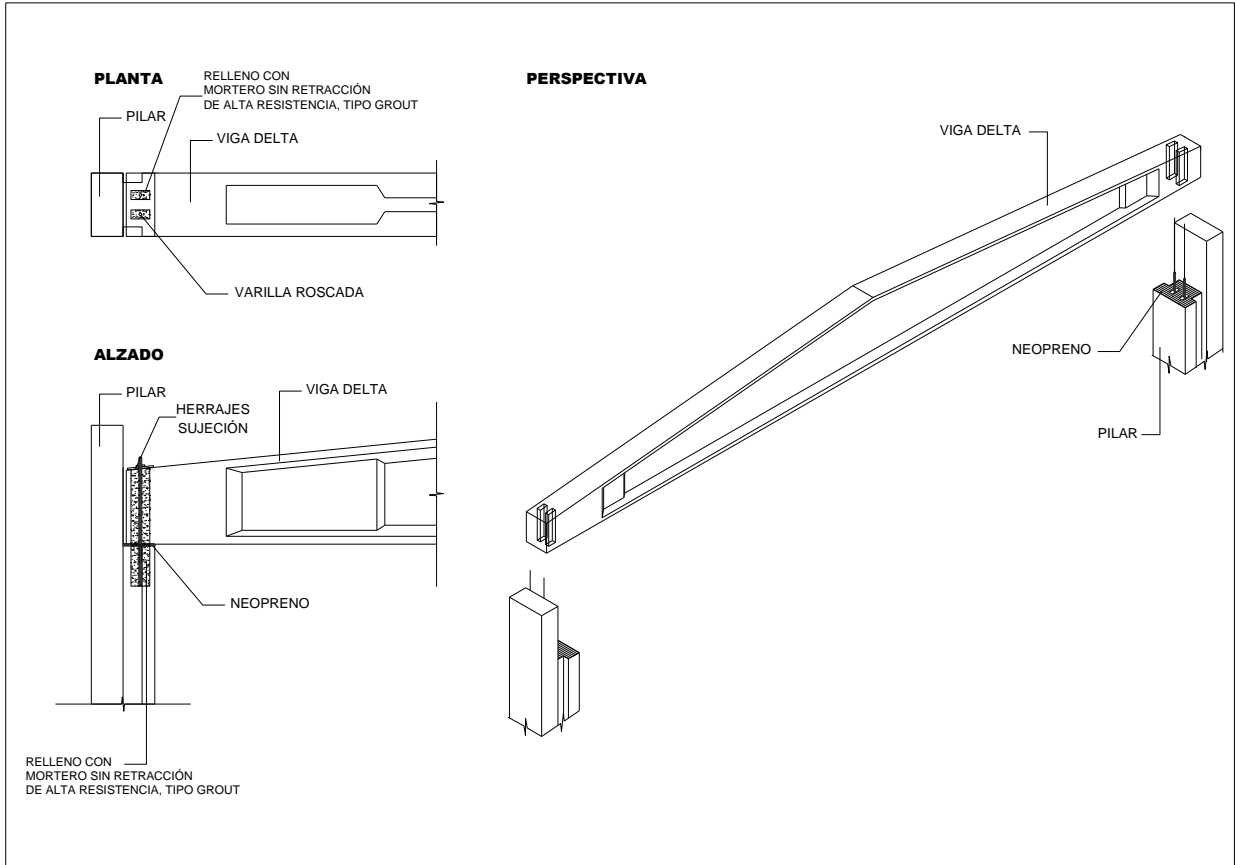
FIGURA 2.6. Unión pilar - viga DELTA para zona sísmica
