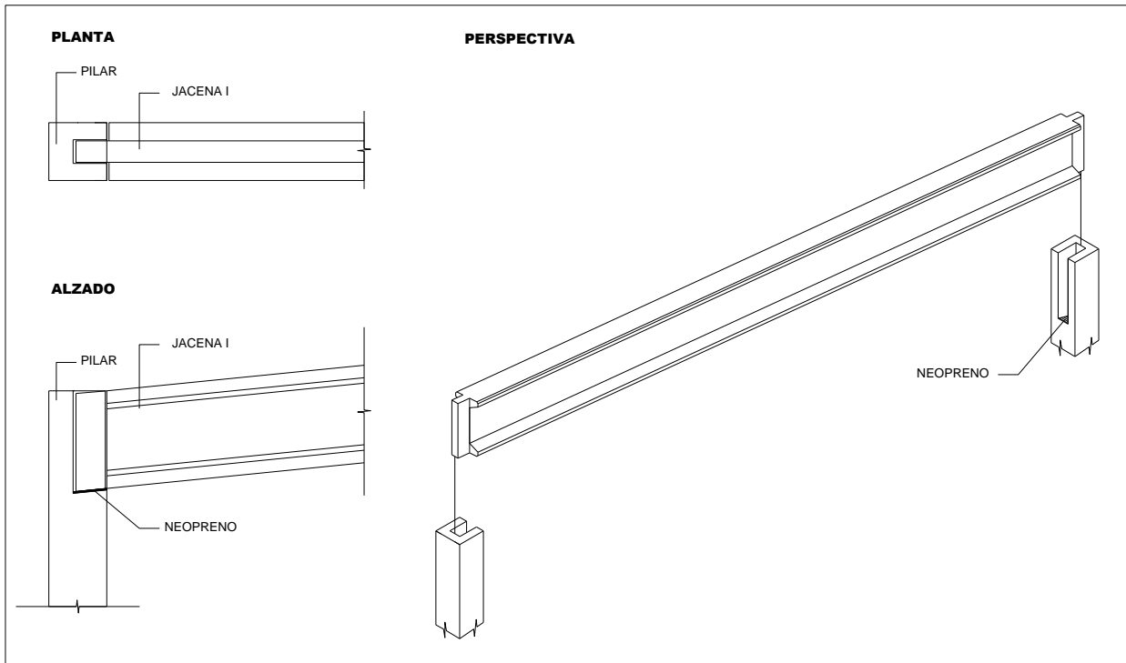
FIGURA 2.1. Unión pilar - jácena tipo
