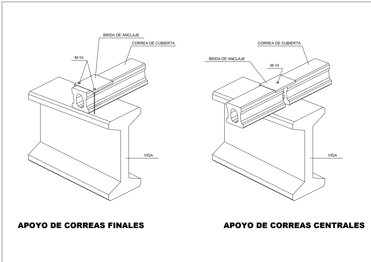
FIGURA 6. APOYOS DE CORREAS
