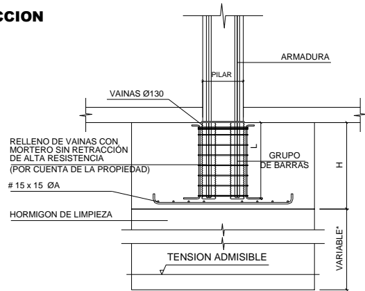
FIGURA 3.2 - UNIÓN MEDIANTE VAINAS
