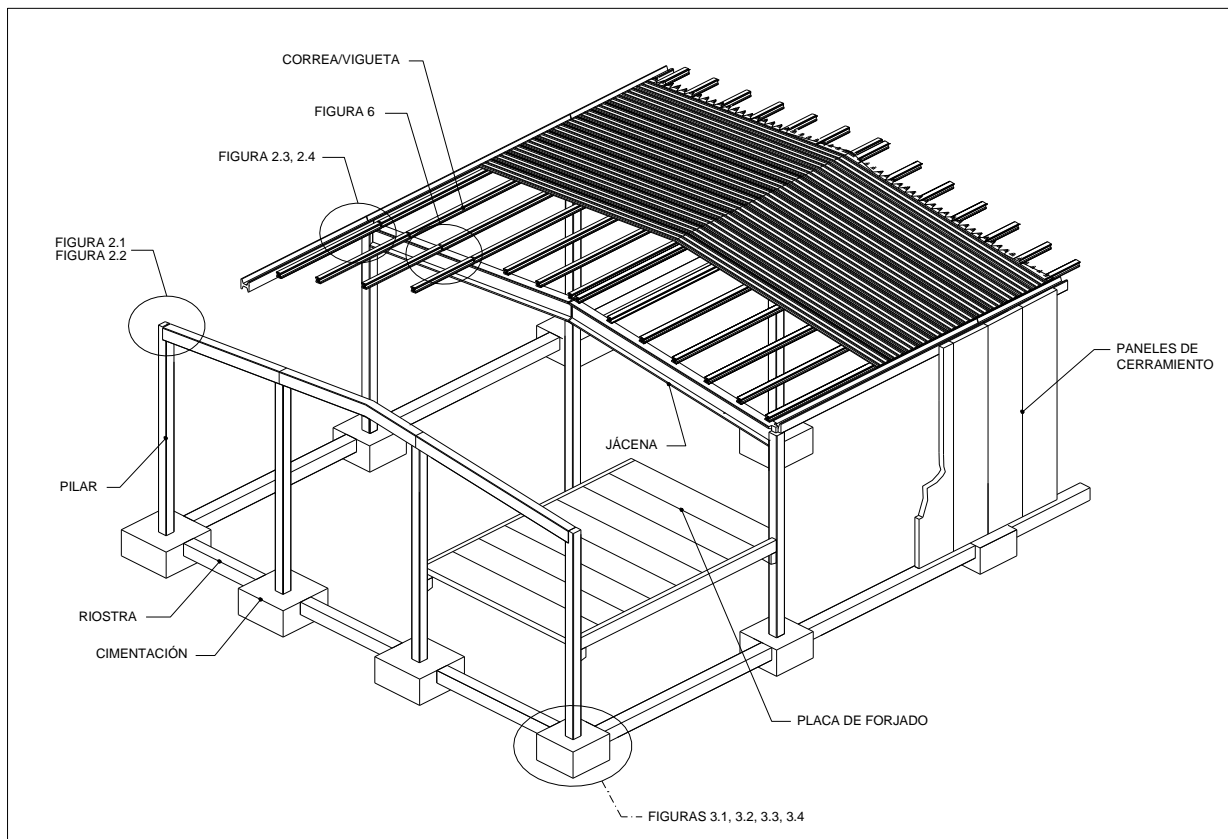
FIGURA 1.2. Esquema general del Sistema JÁCENAS con vigas DELTA
