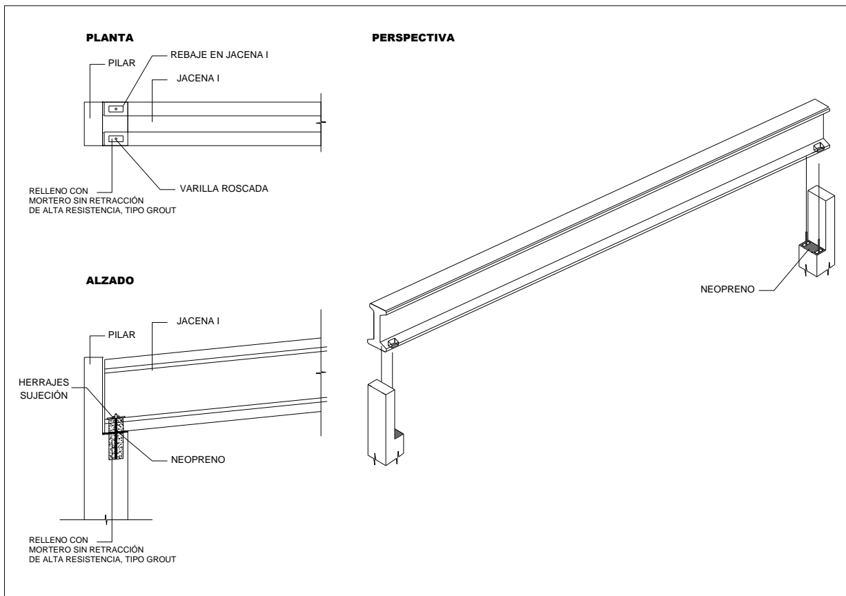
FIGURA 2.2. Unión pilar - jácena tipo I para zona sísmica
