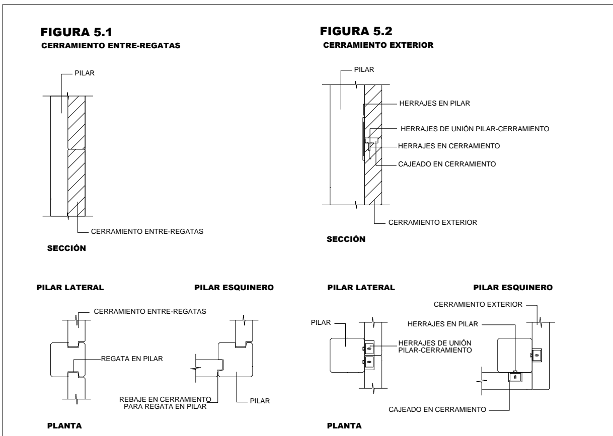
FIGURA 5. UNIONES ENTRE PILARES Y PANELES DE CERRAMIENTO
