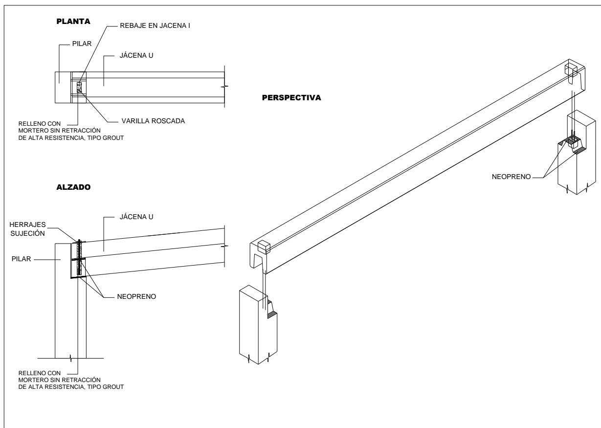
FIGURA 2.4. Unión pilar - jácena tipo U para zona sísmica
