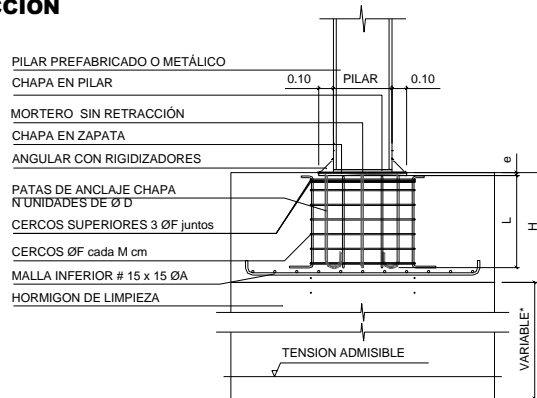
FIGURA 3.4 - UNIÓN SOLDADA
