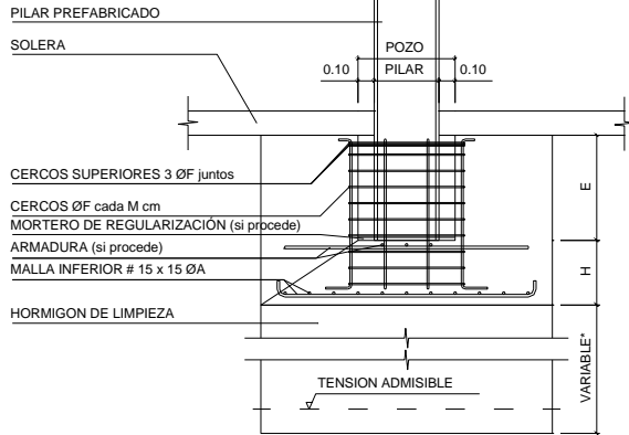
FIGURA 3.1 - UNIÓN MEDIANTE CALIZ
